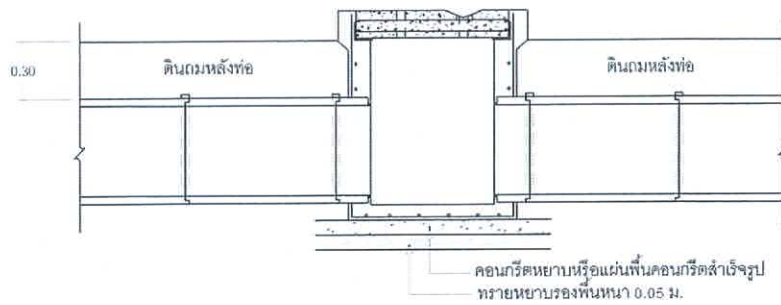
รูปตัด A
