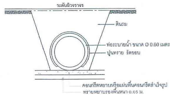
รูปตัด C
